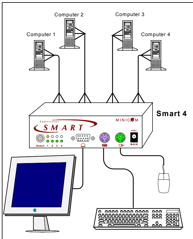
Figura 1 La configurazione Smart 4
